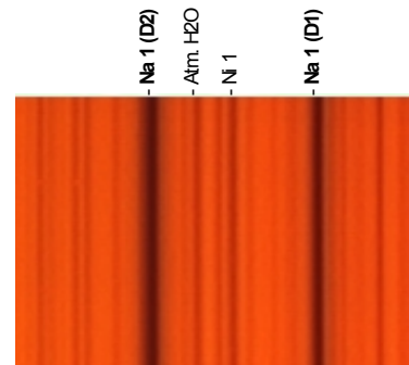
Triplet du Magnésium
