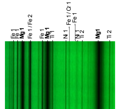
Triplet du Magnésium
